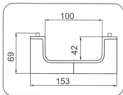
⑥ Лоток Medium B-125 100.65 h85 пластиковый
